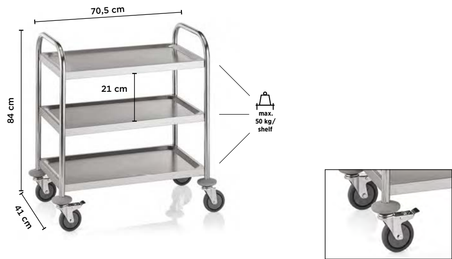
KOLICA ZA POSLUŽIVANJE KARROČË SHËRBIMI SERVING TROLLEY
