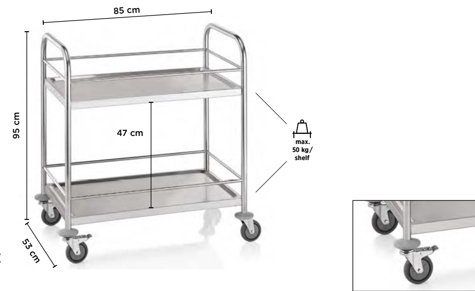
KOLICA ZA POSLUŽIVANJE KARROČË SHËRBIMI SERVING TROLLEY
