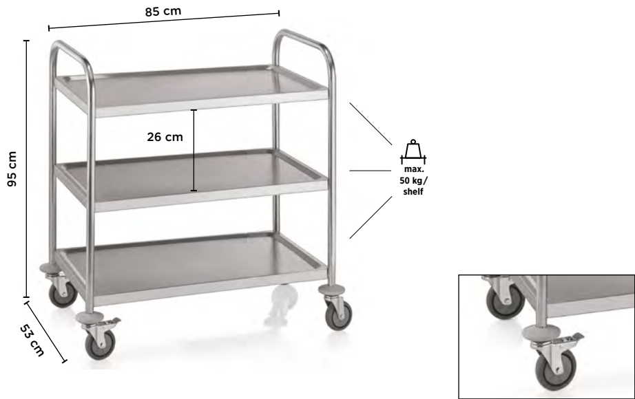
KOLICA ZA POSLUŽIVANJE KARROČË SHËRBIMI SERVING TROLLEY
